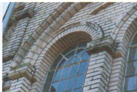
С.Великі Крушлинці, Вінницького р-ну, Вінницької обл. Храм Усікнення голови Іоанна Предтечі. Деталь екстер'єру: цегельна кладка – оздоблення вікон. Листопад 2013р.
